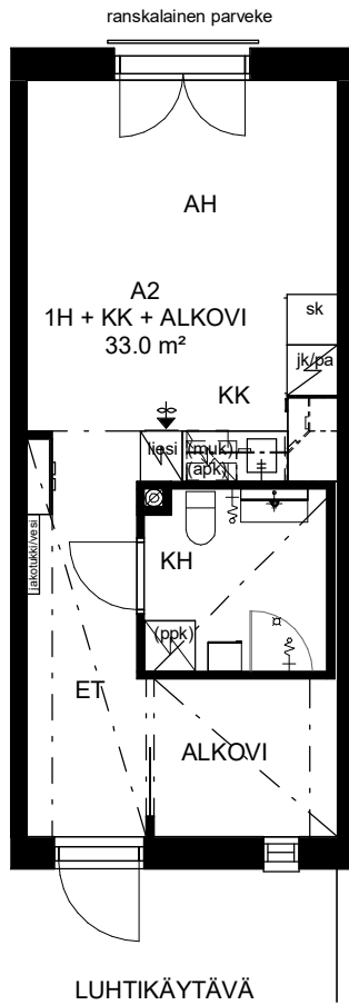
POHJAPIIRUSTUS 1 : 100
