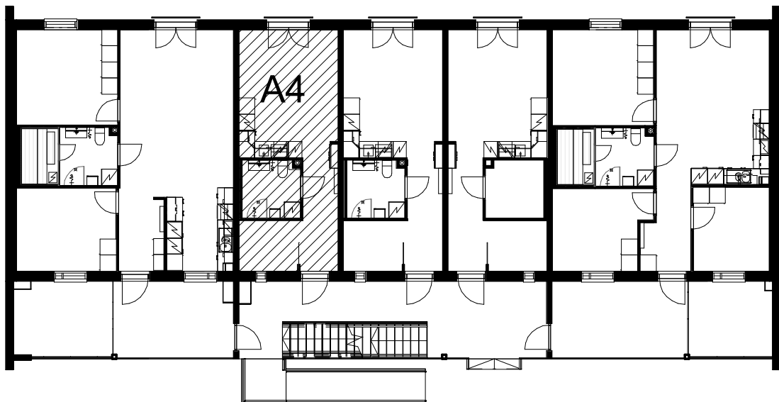
SIJAINTI 1 : 200
