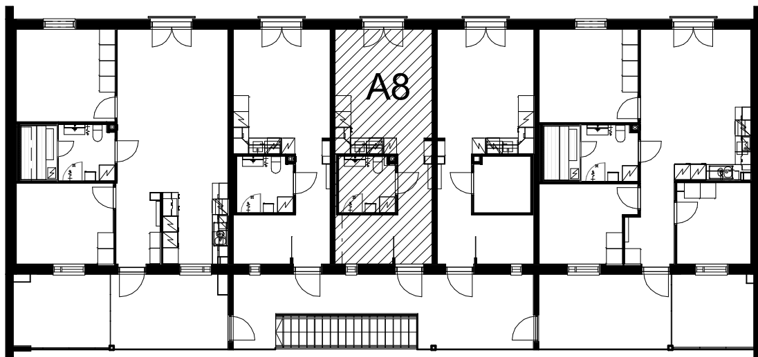
SIJAINTI 1 : 200
