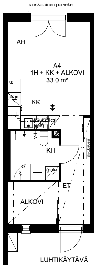
POHJAPIIRUSTUS 1 : 100
